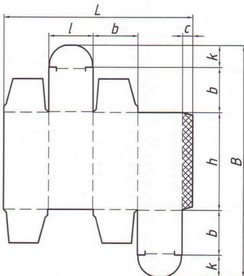
Рис.2. Развертка пачки
