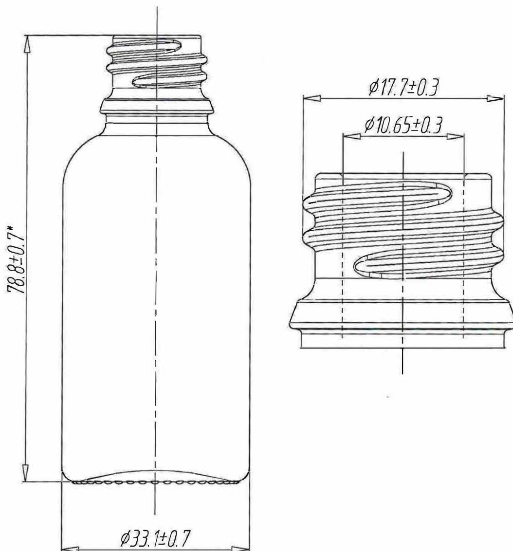
Венчик горловины типа ФК-18
